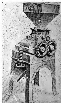
«Richmond & Chandler» Quebradora de maíz
