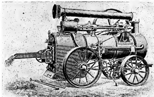
MOTOR LOCOMÓVIL
