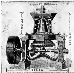
Máquina de romper maíz con marlo
