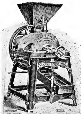
«INKOOS» Máquina de moler maíz
