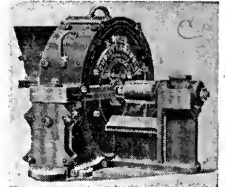
DESINTEGRADORA para moler maíz con marlo ó cualquier otra substancia
