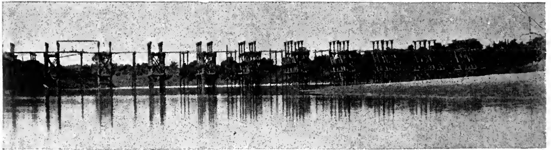
El puente provisional y el andamiaje del definitivo
