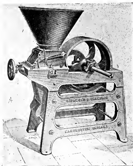
PICADORA DE PASTO
