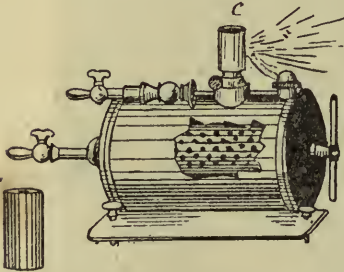
LA LÁMPARA FRES-COURT
