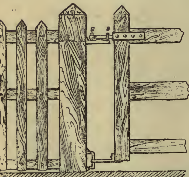
LA BISAGRA APLICADA Á LA TRANQUERA
