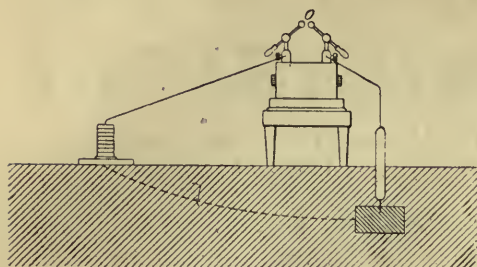
APARATO TRANSMISOR
