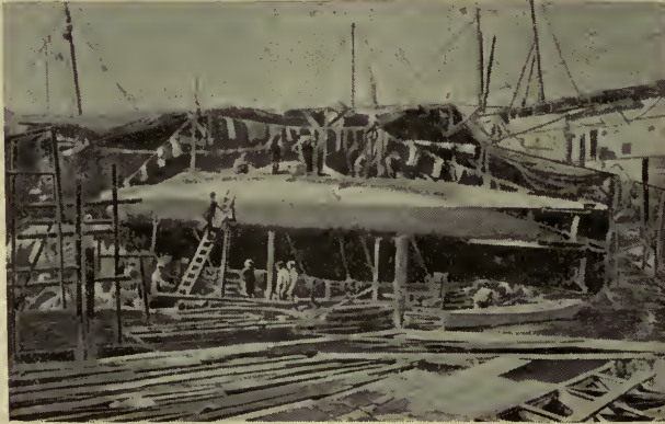
EL «FULTON» LISTO PARA LA BOTADURA
