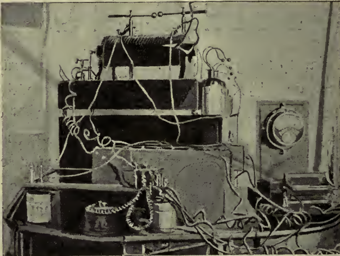
REPETIDOR GUARINI, COLOCADO EN LA TORRE DE S. ROMBAUT, EN MALINAS
