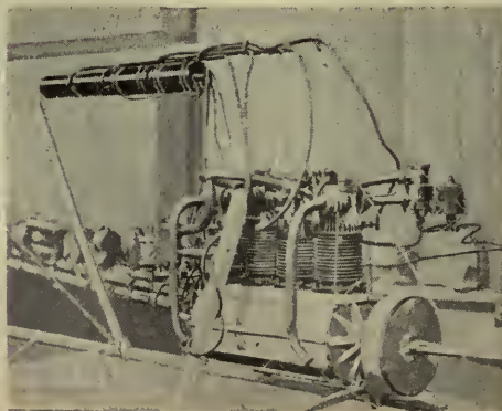
EL MOTOR DEL «SANTOS DUMONT N.º 5»
