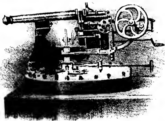
Cañon de repetición argentino, sistema Bollo (privilegiado).
