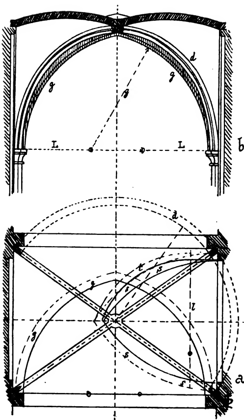
Fig. 101. Gothisches Rippen-Gewölbe.
