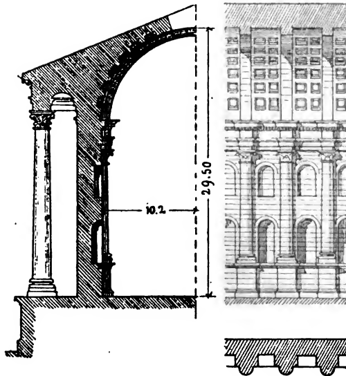
Fig. 91. Aus dem Tempel zu Balbeck. (Römisch.)
