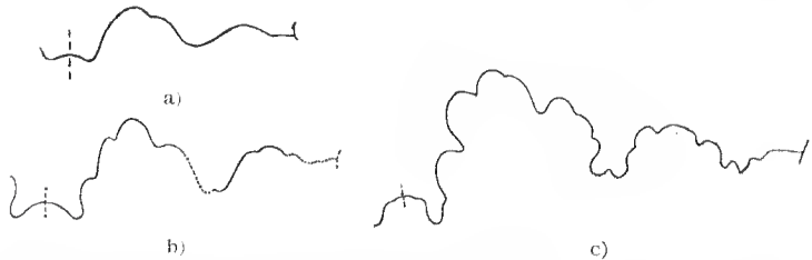
Fig. 23. Entwicklung der Lobenlinie von Acanthoceras ( Pedioceras ?) Jaekeli n. sp. unterhalb Balangli . a) Windungsradius 1 mm, 20/1. b) 4 mm, 10/1. c) 10 mm, 6/1.
