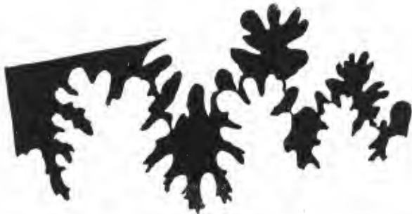
Fig. 70. Barr. cf. Brancoi , Balangi am Mungo. Rechte Sutura. Nat. Gr.
