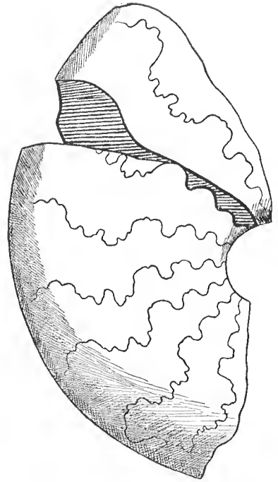
Fig. 34. Lobenlinie von Hopl. ingens costatus (Stück I der Maßstabelle).
