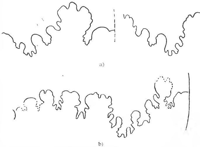
Fig. 41. Lobelinie von Hopl. ingens laevis . (Stück III der Maßstabelle.) a) Erste Lateralloben rechts und links bei 9 mm Windungsradius. 5/1. b) Linke Suture bei 80 mm Windungsradius. Nat. Gr.
