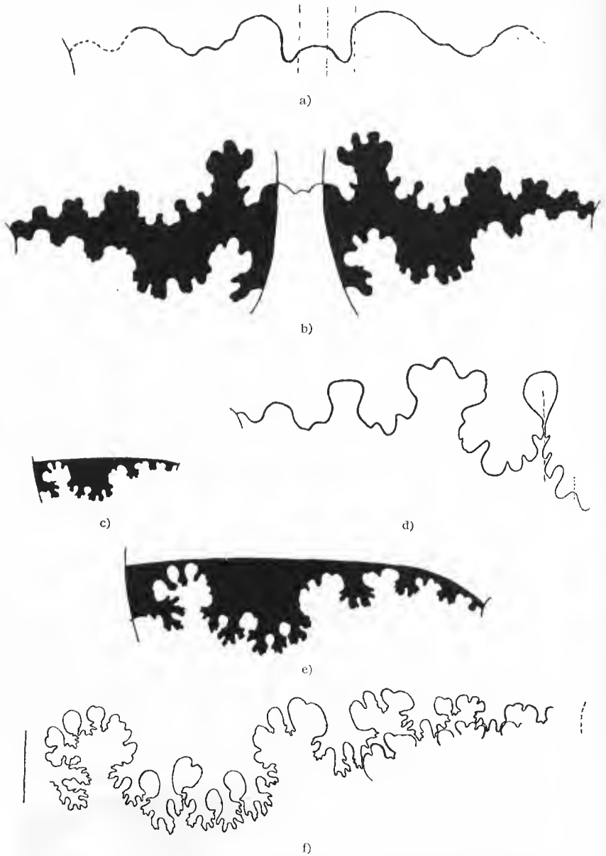
Fig. 40. Lobenlinie von Hopl. ingens laevis (Stück II der Maßtabelle.) a) Sutura bei 3 mm Windungsradius. 15/1. b) Sutura bei 10 mm Windungsradius. 5/1. c) Rechte Sutura bei 14 mm Windungsradius. 2/1. d) Innenloben der rechten Gehäuse- seite bei 14 mm Windungsradius. 10/1. e) Rechte Sutura bei 35 mm Windungsradius. 2/1. f) Rechte Sutura bei 160 mm Windungsradius. 2/3.
