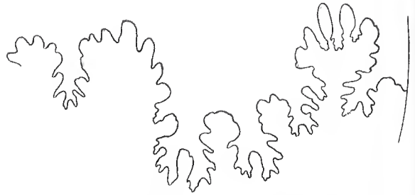
Fig. 25. Linke Sutura (unvollständig) von Hoplitoides Wohlmanni v. K. Elephantenbank (Stück I der Tabelle). Windungsradius 43 mm. 2/l.
