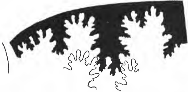
Fig. 63. Suture des auf Taf. V Fig. 4 abgebildeten Stückes (Stück I der Mafstabelle) bei 40 mm Windungsradius.
