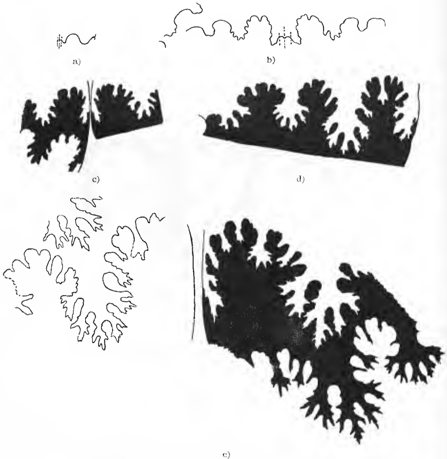
Fig. 17. Entwicklung der Lobenlinie von Neopt. telingaef. var. discrepans n. var. von Balangi. Windungsradius: a) 0,5 mm, 15/l. b) etwa 5 mm, 6/l. c) etwa 15 mm, 4/l. d) 27 mm, 2/l. e) 42 mm, 2/l.
