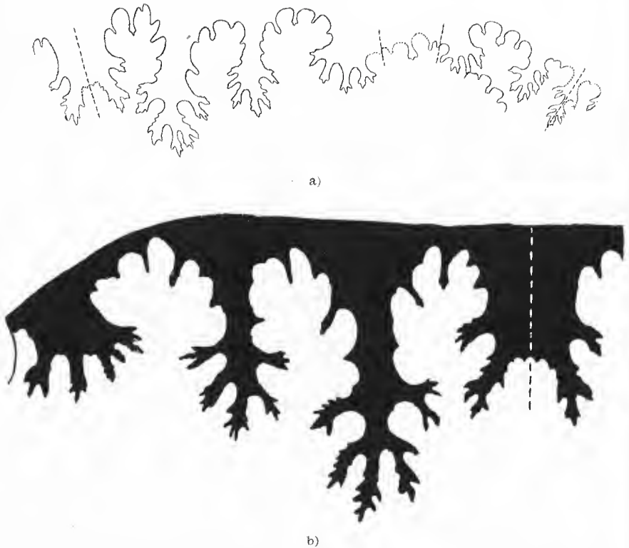
Fig. 18. Lobenlinie von Neopt. crassus n. sp. von Balangi. a) rechte Sutura einschließlich der Innenloben bei 35 mm Windungsradius, 3/2 . b) linke Sutura bei 40 mm Windungsradius, 2/1 .
