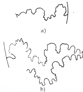
Fig. 43. Lobenlinie von Hopl. Koeneni n. sp. Diki am Mungo. (Stück II der Maßstabelle.) a) Linke Sutur bei 12 mm Windungsradius. 2/l. b) Rechte Sutur bei 18 mm Windungsradius. 2/l.
