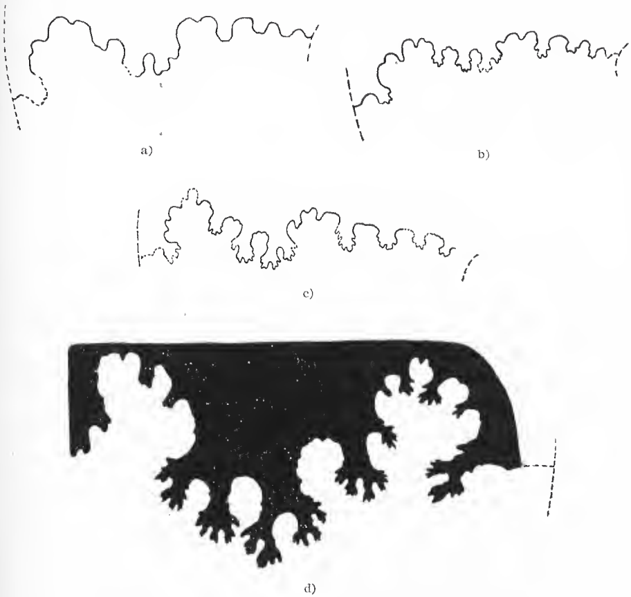
Fig. 31. Lobenlinie von Hopl. ingens nodifer (Stück II der Maßstabelle). a) Rechte Sutura bei 8 mm Windungsradius, 3/1. b) Rechte Sutura bei 15 mm Windungsradius, 4/1. c) Rechte Sutura bei 32 mm Windungsradius, 2/1. d) Erster Laterallobus links bei 90 mm Windungsradius, 3/2.
