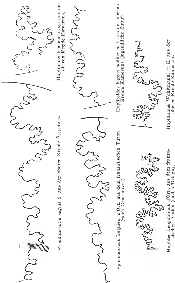
Fig. 74. Konvergente Entwicklungen der Lobenlinie.
