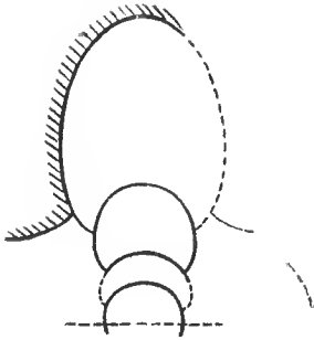
Fig. 24. Querschnitt der Jugendwindungen von Hoplitoides Wohlmanni v. K. Elephantenbank (Stück II der Tabelle). 10/l.
