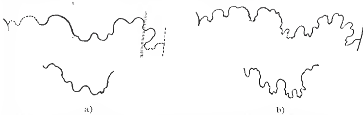
Fig. 42. Lobenlinie von Hopl. Koeneni n. sp. Elefantbank am Mungo. (Stück I der Maßstabelle.) a) Linke Sutur und erster Laterallobus der rechten Sutur bei 4 mm Windungsradius. 10/l. b) Desgl. bei 23 mm Windungsradius. 2/l.
