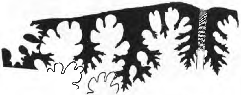
Fig. 11. Lobenlinie von Neopt. telingaef. n. sp. (von dem in Taf. III Fig. 2 abgebildeten Stück). a) rechte Suture bei 20 mm Windungsradius 2/1 . b) linke Suture bei 15 mm Windungsradius 2/1 .
