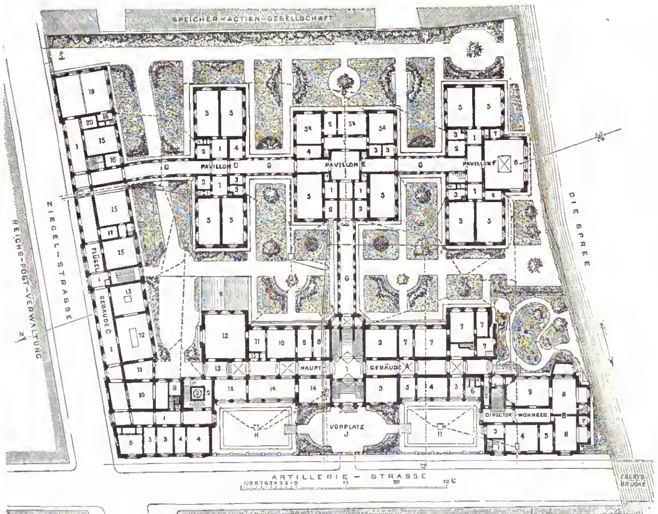
Situationsplan des geburtshilflichen Klinikums.
