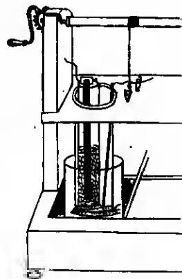
Schema zur Tauchvorrichtung. Grösse und Anzahl der Elementenreihen können beliebig gewählt werden.
