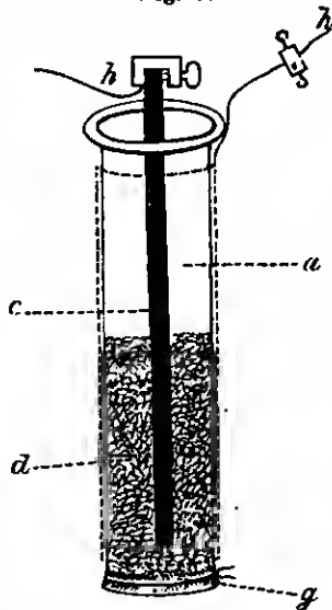
a äusserer, h innerer Cylinder, c Kohlenplatte, d Braunstein-Kohlegemenge, e Zinkplatte, f Leinwandboden des inneren Cylinders, g Leinwandboden des äusseren Cylinders, h Leitungsdrähte und Klemmen für Kohlen- und Zinkplatte. Die punctirten Linien bezeichnen den über den Glaszylinder zu schiebenden Zinkcylinder.
