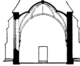
Längenschnitt 1 : 400 Querschnitt nach Aufnahme von Tappe.
