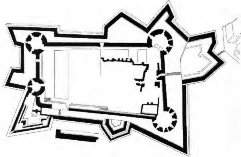
Grundriß 1 : 2500. Nach einer Aufnahme im Besitze des Kriegsarchivs zu Berlin.
