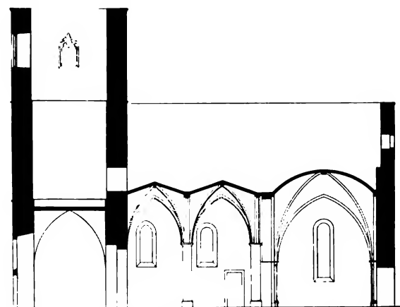
Längenschnitt
