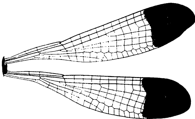
Fig. 102.—Wings of Chloroneura apicalis Fras., male.
