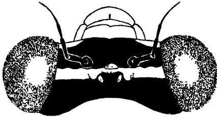
Fig. 93.—Head of Copera superplatypes Fras., male.
