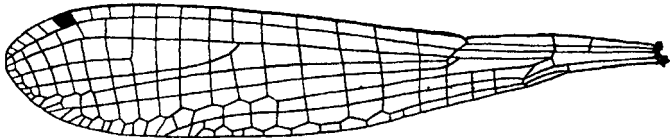
Fig. 129.—Wing of Archibasis mimetes præclara (Fras.), male.
