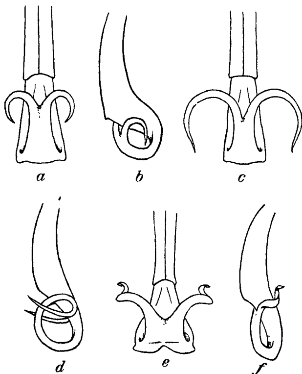
Fig. 46.—Penile organs of:—a & b. Rhinagrion mima (Karsch); c & d. Mesopodagrion tibetanum MacL.; e & f. Burmargiolestes melanothorax (Selys).
