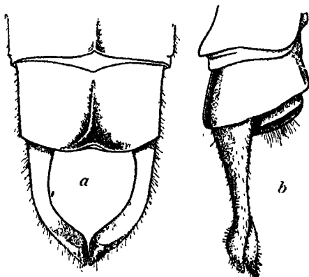
Fig. 43.—Anal appendages of Rhinagrion mima (Karsch), male. a. Dorsal view. b. Right lateral view.
