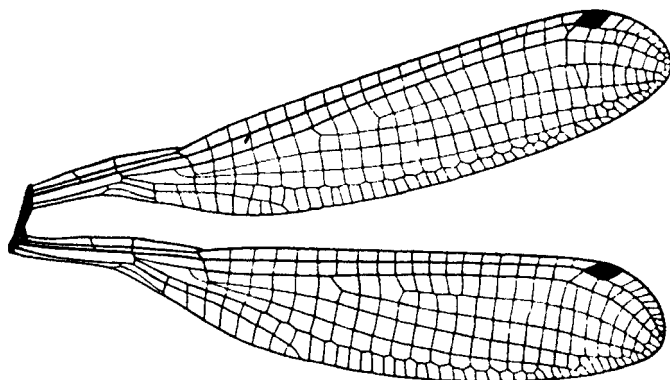
Fig. 111.—Wings of Esme cyaneovittata Fras., male.
