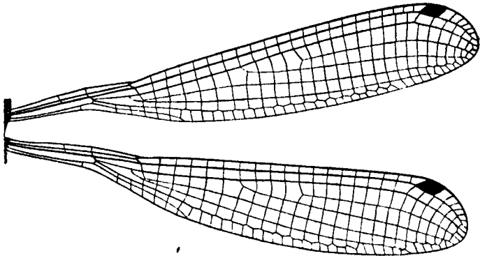
Fig. 109.—Wings of Melanoneura bilineata Fras., male.
