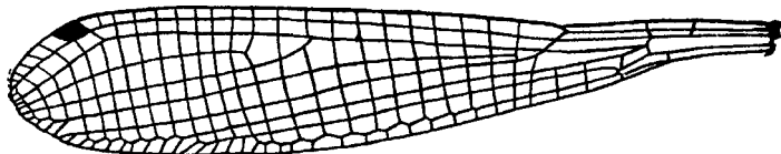
Fig. 71.—Wing of Cæliccia membranipes (Ramb.), male.
