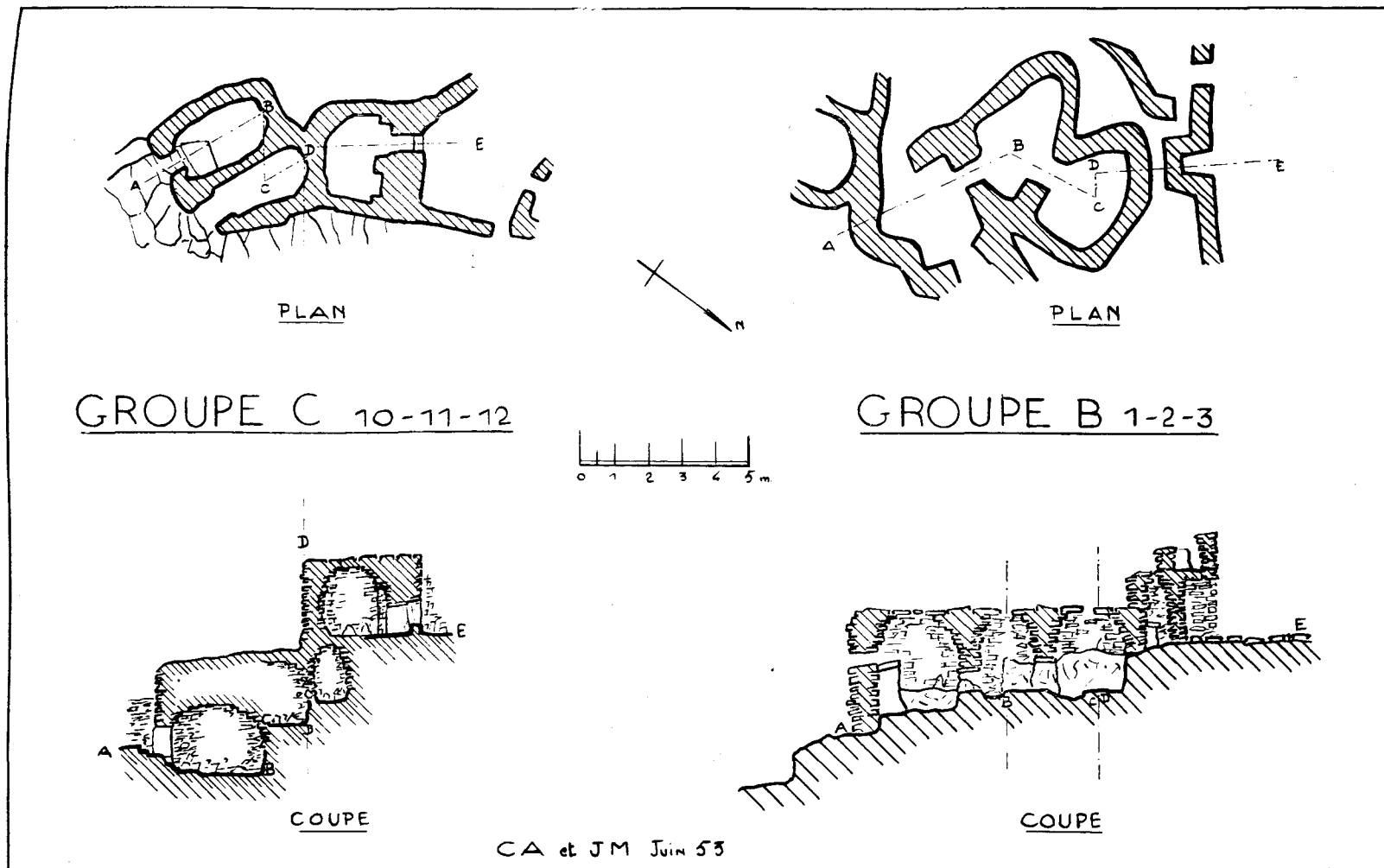
Fig. 4. — Jebel Lakhdar. Coupe dans 2 groupes d'habitations.
