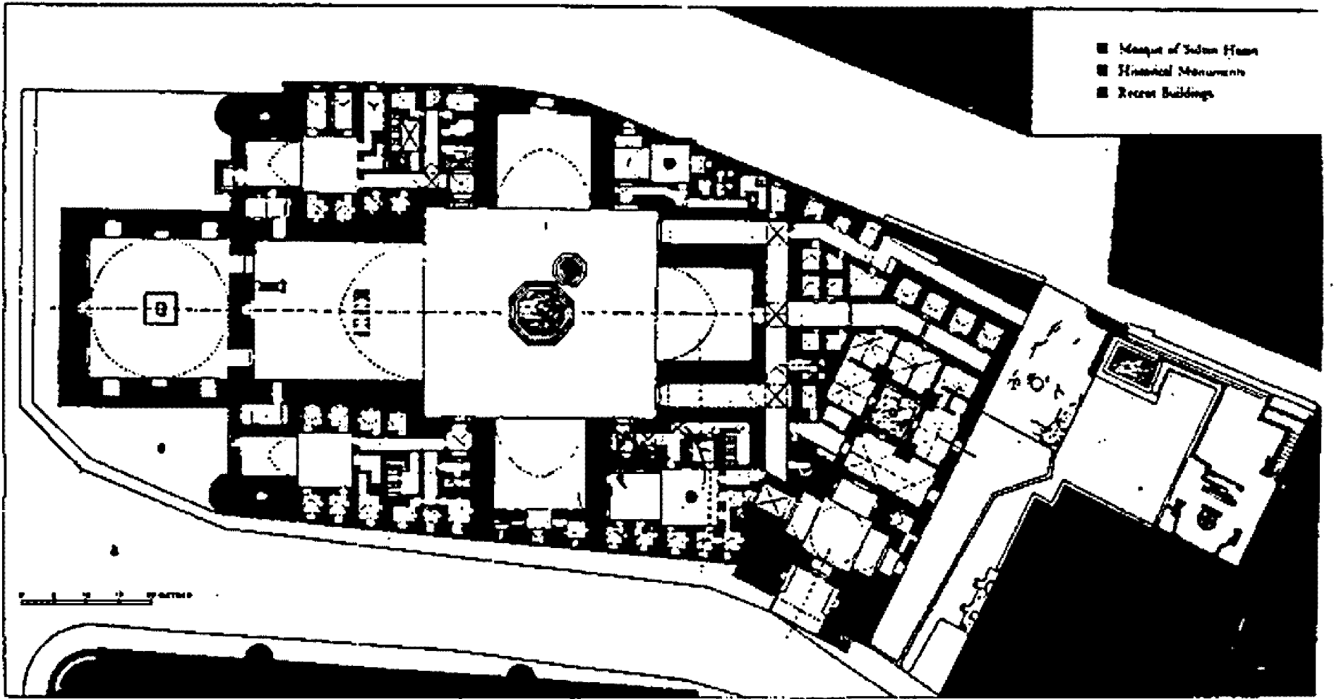
خطة جامع ومدبرة السلطان حسن المصدر : كروسويل ، ام . اي . اي ، الجزء الأول شكل ٦٦
