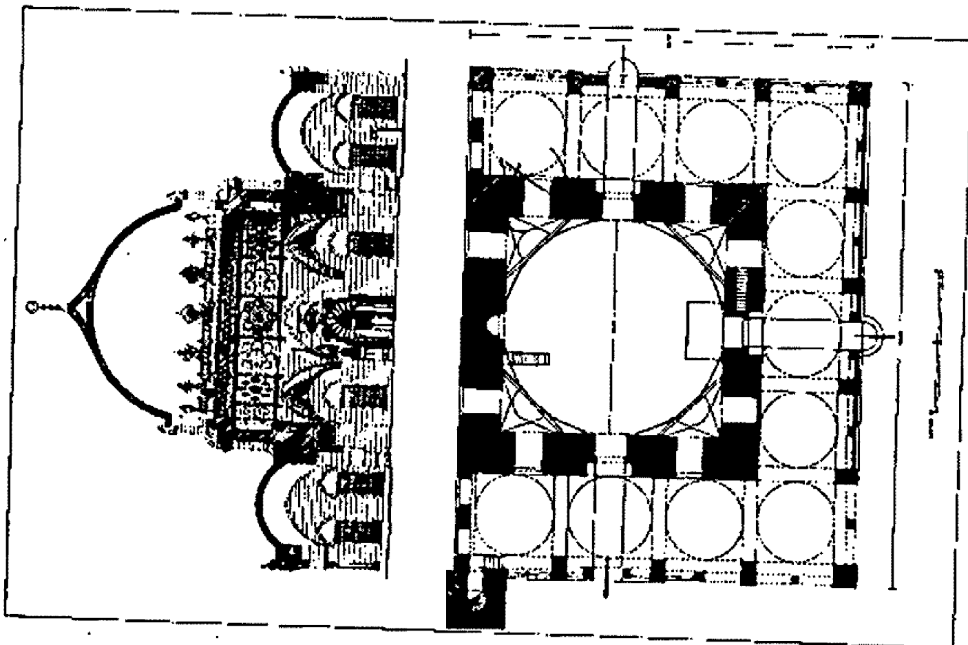
خطة وارتفاع جامع سلطان حسن م ٩٧٩ / ١٥٧٦ م المصدر : كروسويل ، ام . اي . اي ، الجزء الثاني شكل ١٠٩ ، ١١٠
