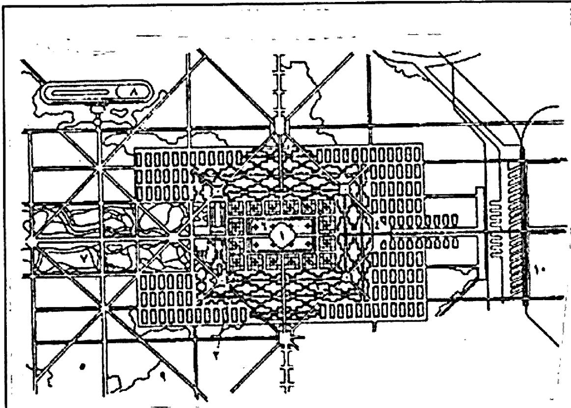
المخطط التصميمي لمدينة تسع لثلاثة ملايين نسمة، وقد وضعه المهندس المعماري لي كوربوزيه محطة، ٢. ناطحة سحاب، ٣. قطع اراضي ذات نوات بارزة، ٤. قطع ارضية مغطاة، ٥. مناطق المدينة الحدائقية، ٦. بنايات عامة، ٧. للحديقة الانجليزية، ٨. ساحة سباق الخيل، ٩. منطقة احتياطية، ١٠. لهواض السفن، ١١. مركز صناعي ومحطة للبضائع.
