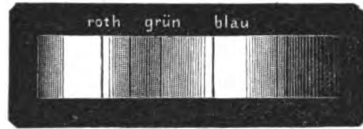
Absorptionsspectrum des violetten Manganglases.
