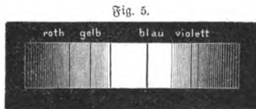
Spectrum des durch dunkelblaues Kobaltglas gegangenen Lichts.
