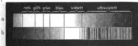
a Sonnenspectrum, b Photographie des Sonnenspectrums.
