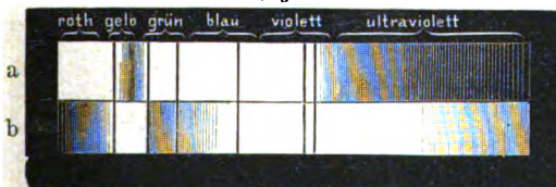
a Sonnenspectrum, b Photographie desselben mittelst anilinroth gefärbter Platte
