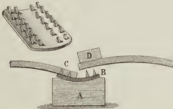
FIG. 111. Riemen Clip.
