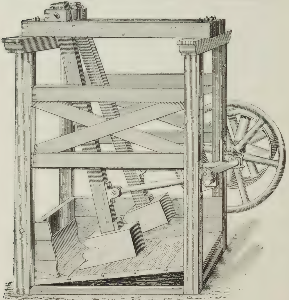
FIG. 83.—“Stocking” machine.
