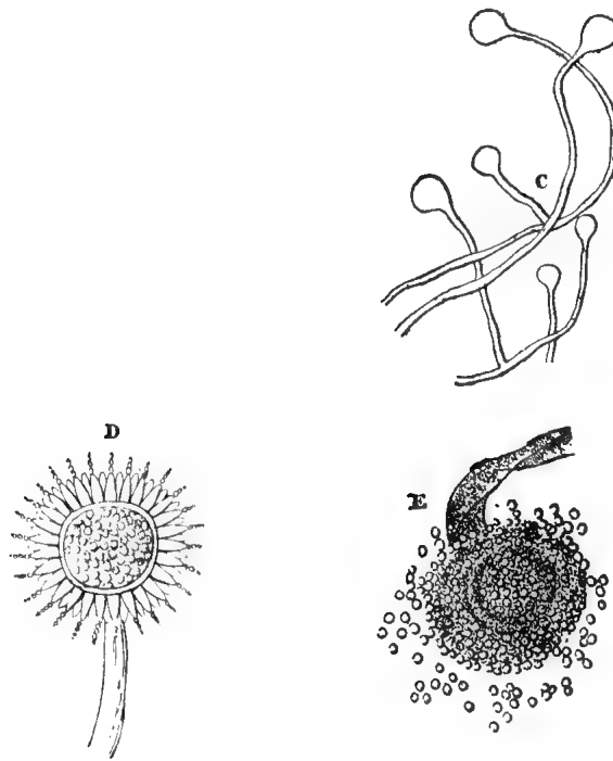
FIG. 6.— Aspergillus Niger .
