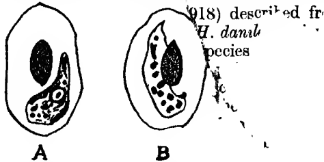
Fig. 109.— Haemoproteus herodiadis de Mello.
