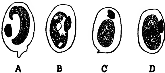
Fig. 110.— Haemoproteus kopki (de Mello).
