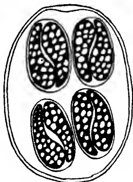
Fig. 97.— Eimeria yakimovi Rastegaïeff. (After Rastegaïeff.)
