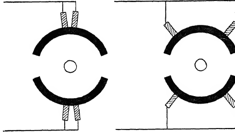
FIG. 92.—Double-brush rectifier.
