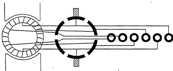
FIG. 122.—Leblanc's Panchahuteur.
