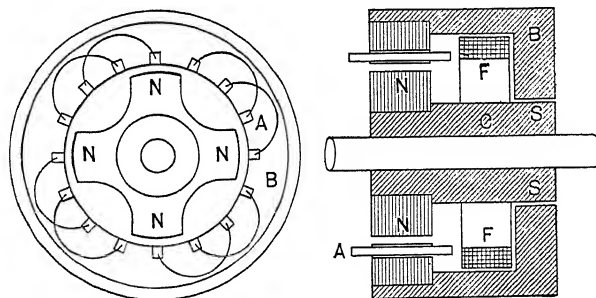
FIG. 136.—Inductor alternator.
