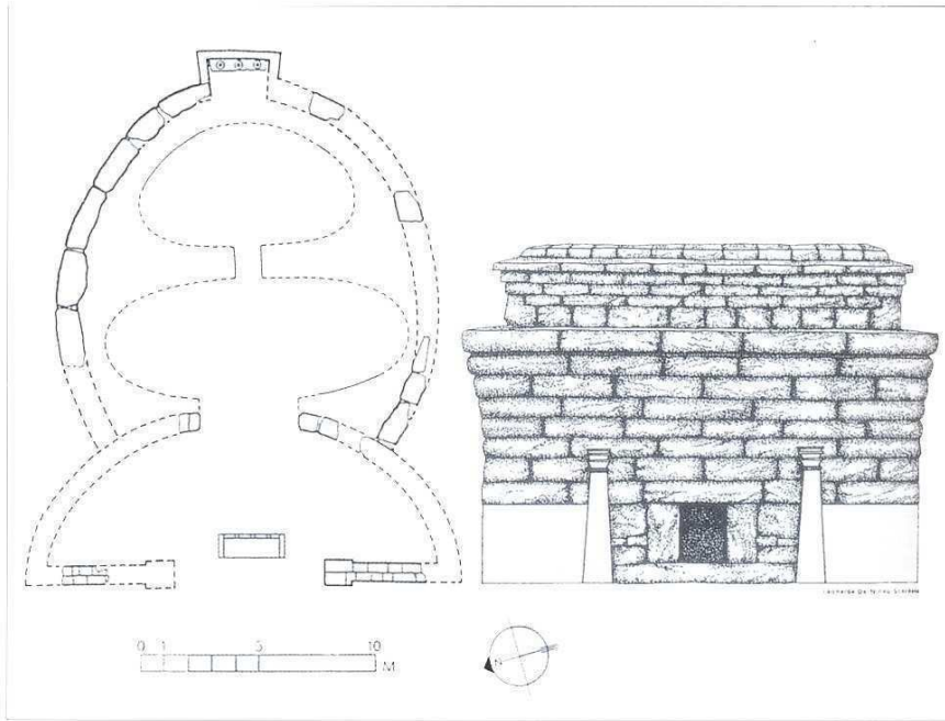
Fig. 8: Ricostruzione del tempio nella sua fase fenicio-punica in pianta ed in alzato della facciata. (Bruno 2004: 106 fig. 23, rielaborata da Ciasca 1976-1977 e id. 1999)
