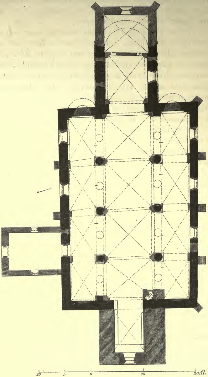
Grundplan af Tandrups Kirke (1873).
