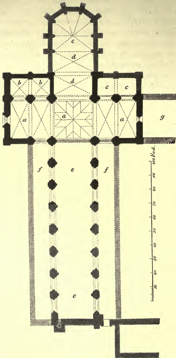
Fig. 8. Plan af Klosterkirken i Colbaz.
