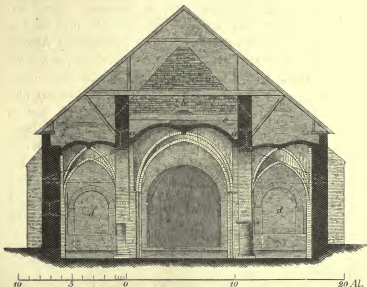
Fig. 4. Tværsnit af Langhuset set imod Koret.
