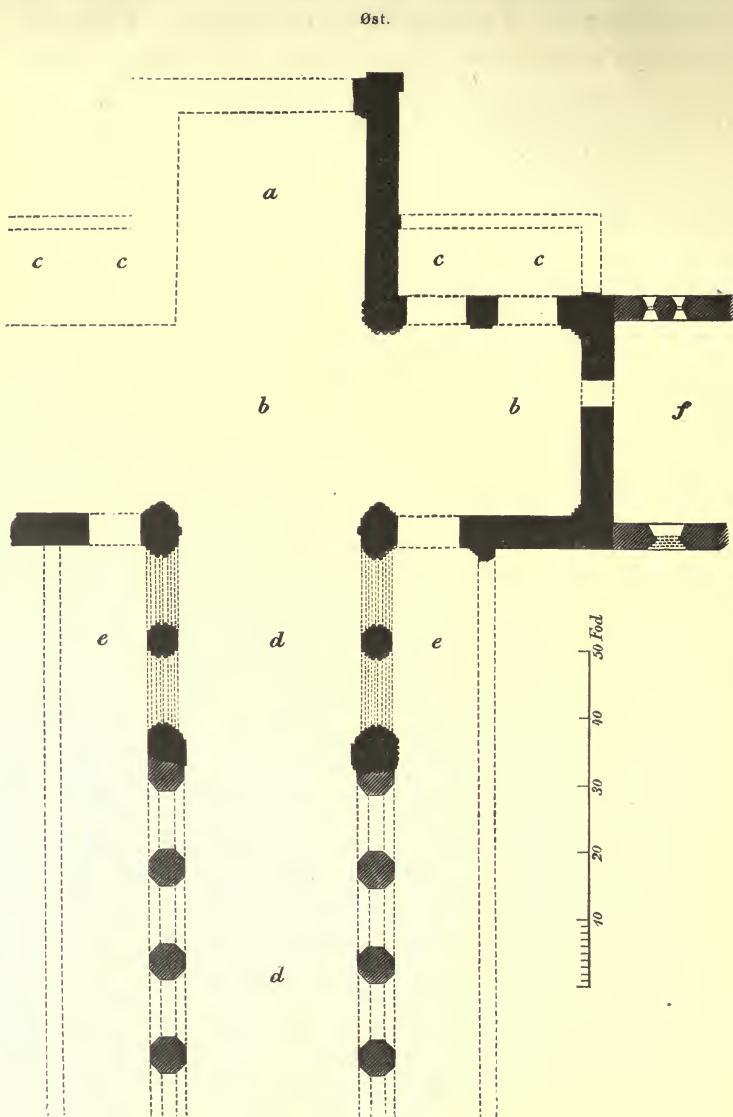
Fig. 4. Plan af den ældre Del af Hilda Klosterkirke.
