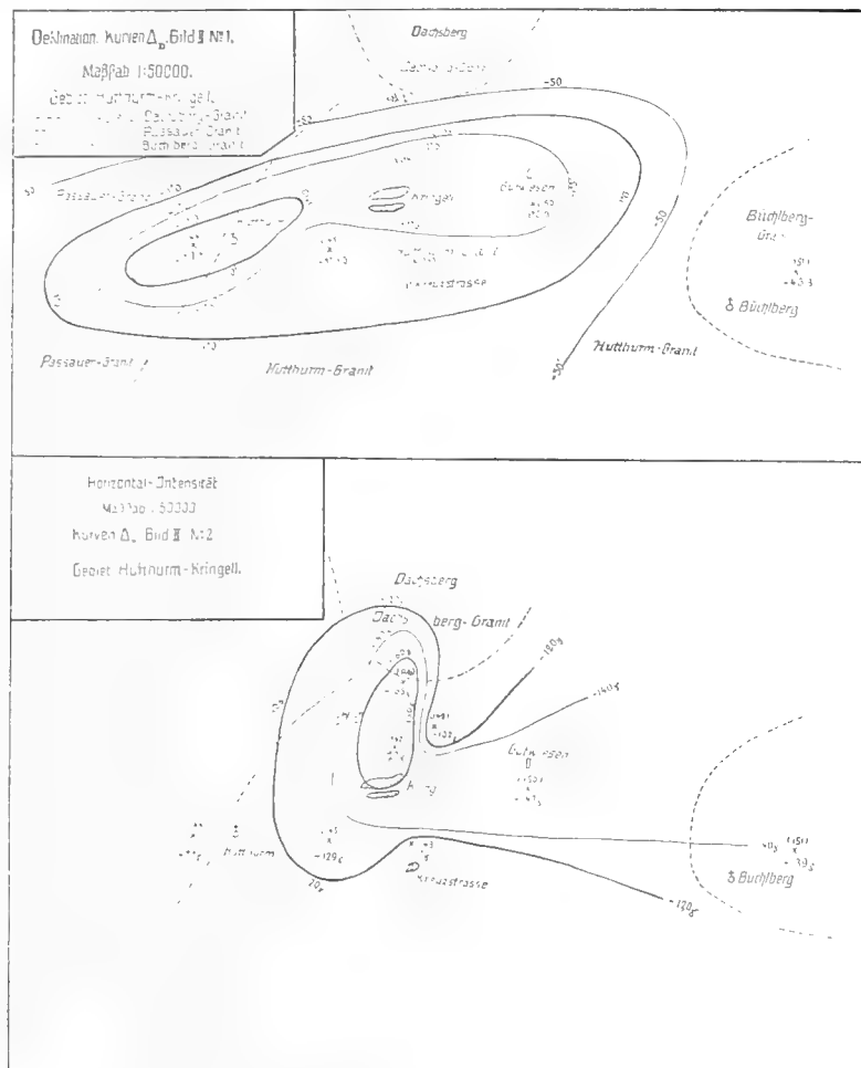
Bild II. Gegend Dachsberg-Hutthurm-Kringell. No. 1. Deklination. Verlauf der \Delta_D -Kurven. No. 2. Horizontalintensität. Verlauf der \Delta_H -Kurven.
