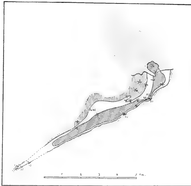
Abb. 14. Geologische Kartenskizze des Muldenzeugen Hefhuf (60 m hoch): außen Hornsteindolomit, mitten Sandsteine und Kalke, innen Knochenbett und hangende Kalke, im N Basalt. 1:125000.
