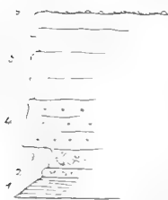
Abb. 4. Übergreifen von Untereocän auf dem Gebel Qasa. 1 helle Cenomantone (bis 37 m über dem Hauptsandstein), 2 Brekzie aus Esogyra Rouvillei des Cenoman, 3 Cenomanton mit Kalkkonkretionen und Geröllen, 4 Kalk mit Nummulites Ramondi , Löchern und Geröllen 5 gelber dolomitischer Kalk mit zahlreichen eocänen Fossilresten, 6 Brocken des gelben Kalks und Flugsand. 1:400.
