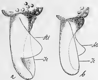
Fig. 4. Achorutes armatus Nic. Mucro: a) Aussen-, b) Innenansicht, von der Seite gesehen. Al Aussenslamelle, Il Innenlamelle. × 1200.
