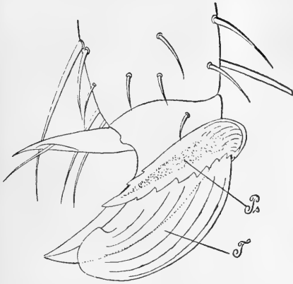
Fig. 38. Sminthurus fuscus (L.) Tullb. Distales Tibienende, Tarsus und Klauen des 1. Beinpaares, Seitenansicht. Ps Pseudonychien, T Tunica. × 500.
