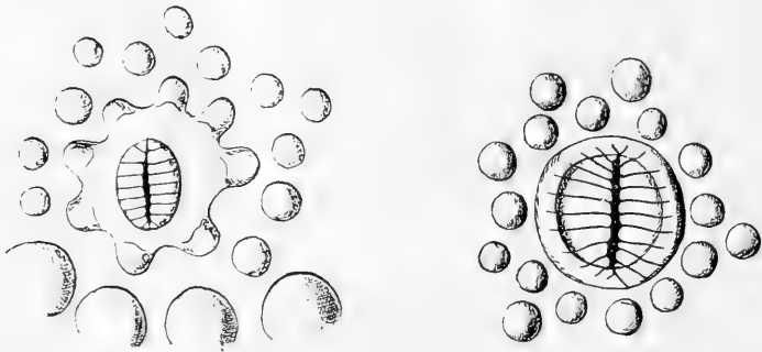
Fig. 6. Aphorura tuberculata (Mon.). Pseudocelle. \times 2400 . Fig. 7. Aphorura armata (Tullb.). Pseudocelle. \times 2400 .
