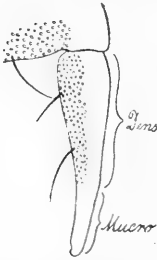
Fig. 2. Furca von Xenylla maritima Tullb. × 500.
