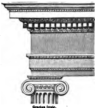
Grecian Ionic.
