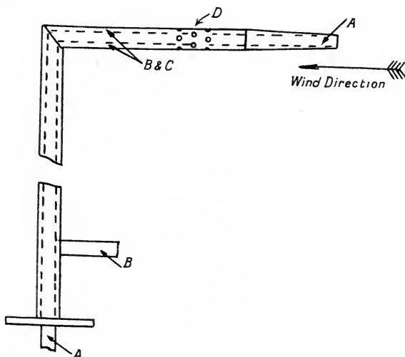
FIG. 1.—Pitot tube.
