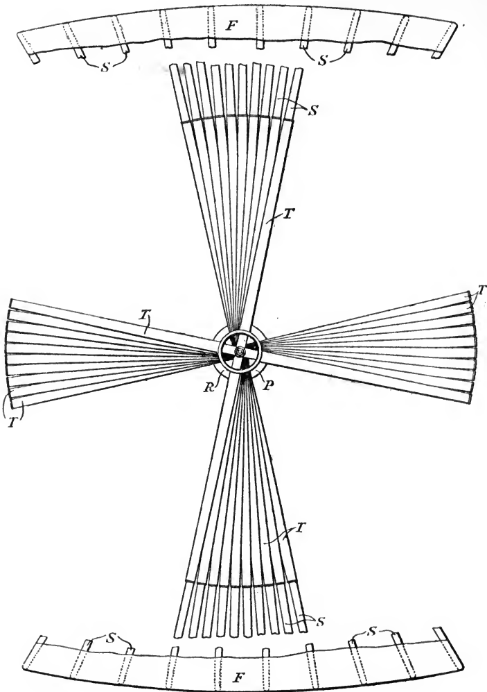
Fig. 5.—Maxim's Propeller.
