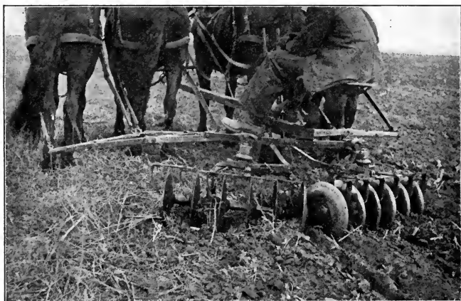
FIG. 266. THE DISK HARROW
