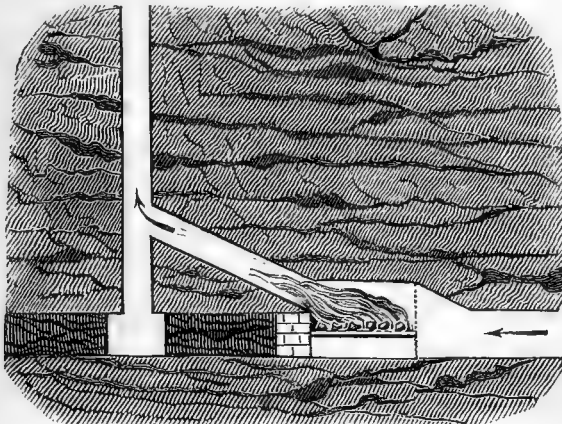
Fig. 13. LUCHTVERVERSINGSOVEN.
