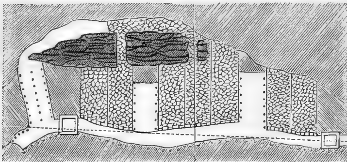
Fig. 4. BEWERKING DOOR DWARSANGANGEN.
