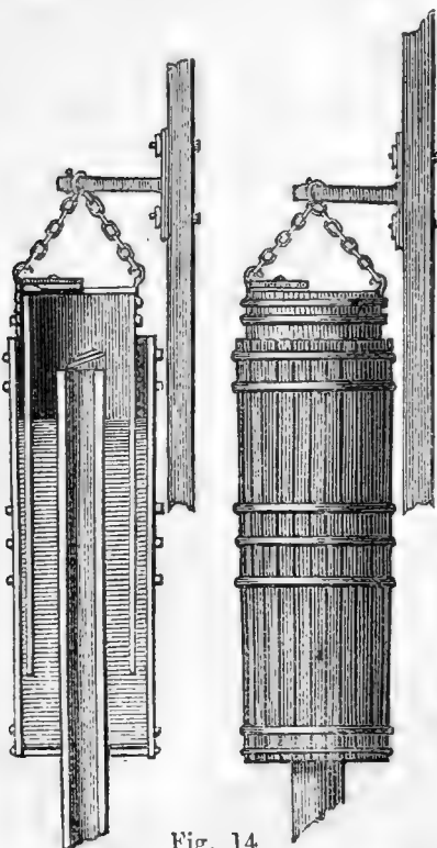
LUCHTVERVERSCHINGSWERKTUIG.
