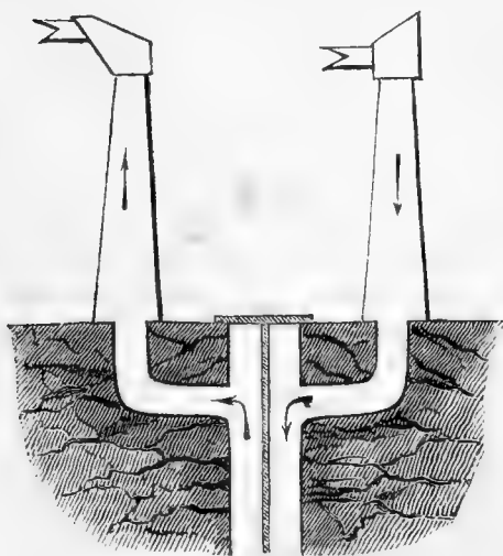
Fig. 11. LUCHTVERSCHING DOOR EEN PUT MET SCHOORSTEENEN.
