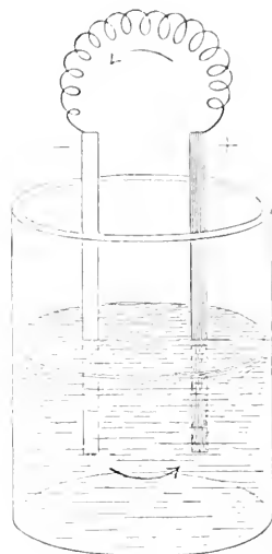
Fig. 188. Galvanisches Element. Der freie Zinkpol (–) ist mit dem freien Kupferpol (+) durch einen Draht verbunden, so dass ein Stromkreis entsteht, in dem die Richtung des Stromes durch die Pfeile angegeben ist.
