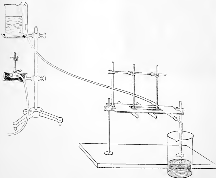
Fig. 228. Apparat zur Untersuchung der Thermotaxis. Auf einer Metallplatte befindet sich, in eine Vertiefung eingelassen, eine flache Wanne aus schwarzem Ebonit (Fig. 227), in der die paramoecienhaltige Flüssigkeit ist. Die Metallplatte besitzt 3 Röhren, durch die von einem Becherglase aus mittels eines Schlauches Wasser von beliebiger Temperatur hindurchgelassen werden kann. Ueber der Wanne sind an einem Stativ Thermometer angebracht, die in die paramoecienhaltige Flüssigkeit tauchen und es gestatten, die Temperatur, die hier an verschiedenen Stellen herrscht, jeden Augenblick abzulesen. Nach MENDELSSOHN.
