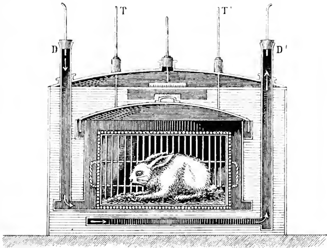
Fig. 117. DULONG'S Wassercalorimeter. Kasten mit doppelter Wand. In dem breiten Raume zwischen beiden Wänden befindet sich Wasser, durch das in Schlangenwindungen ein Rohr nach dem Innern des Kastens läuft, um von aussen her bei D dem Thiere, das sich im Kasten befindet, Luft zuzuführen und die verbrauchte Luft durch D' wieder abzuführen. Bei T u. T' befinden sich Thermometer. Nach ROSENTHAL.
