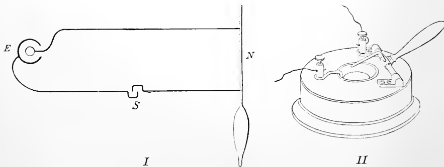
Fig. 190. I Stromkreis, abgeleitet von dem Element E zu dem Nerven N eines Nervemuskelpräparats. Im Stromkreis befindet sich der Schlüssel S. II Quecksilberschlüssel.
