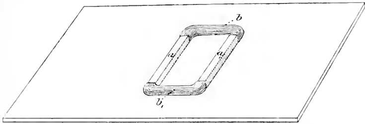
Fig. 197. Objectträger mit Kästchen für galvanische Reizung mikroskopischer Objecte. a und a' , Leisten von gebranntem Thon, b und b' , isolirende Kittwälle, welche mit den Leisten zusammen ein Kästchen abgrenzen, in das die Objecte gebracht werden.
