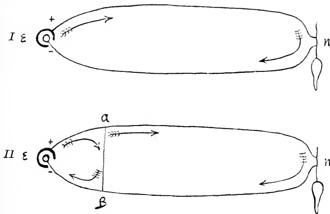
Fig. 192. Princip der Nebenschliessung. I Ein einfacher Stromkreis, II Stromkreis mit Nebenschliessung. E Element, N Nervenmuskelpräparat, A B Nebenschliessung.
