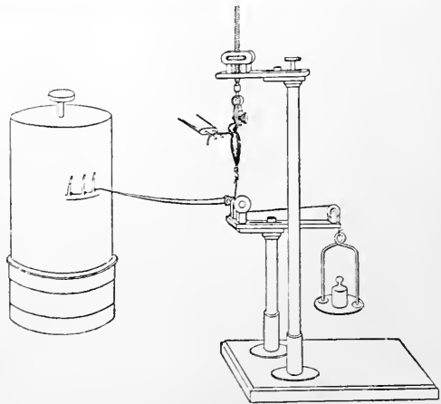
Fig. 205. I Myographion. II Zuckungcurve. Nach HELMHOLTZ. a Moment der Reizung durch einen Inductionsschlag.
