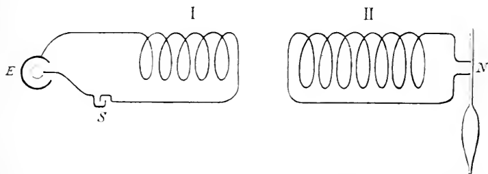
Fig. 194. Inductionsstrom. I Primäre Spirale. E Element, S Schlüssel. II Secundäre Spirale. N Präparat.
