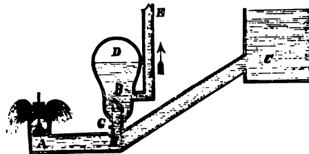
FIG. 1.—Hydraulic Ram.
