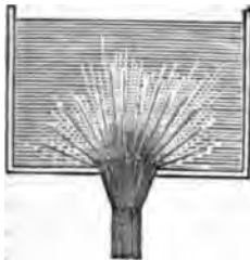
FIG. 18.—Vena Contracta.
