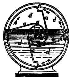
Fig. 9.—Gas Meter.
