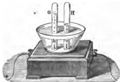
FIG. 24.—Voltmeter.
