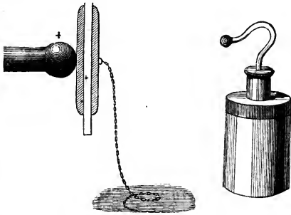
Fig. 16.—Leyden Jar.
