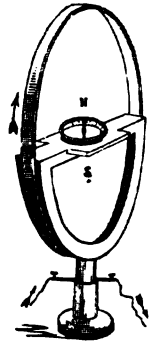
FIG. 18.—Tangent Galvanometer.
