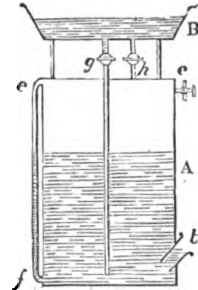
FIG. 3.—Gas-holder.
