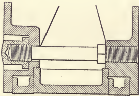
Fig. 69. Sweets' flower bolt.
