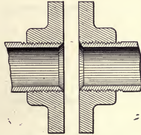
Fig. 21. Peened Joint.
