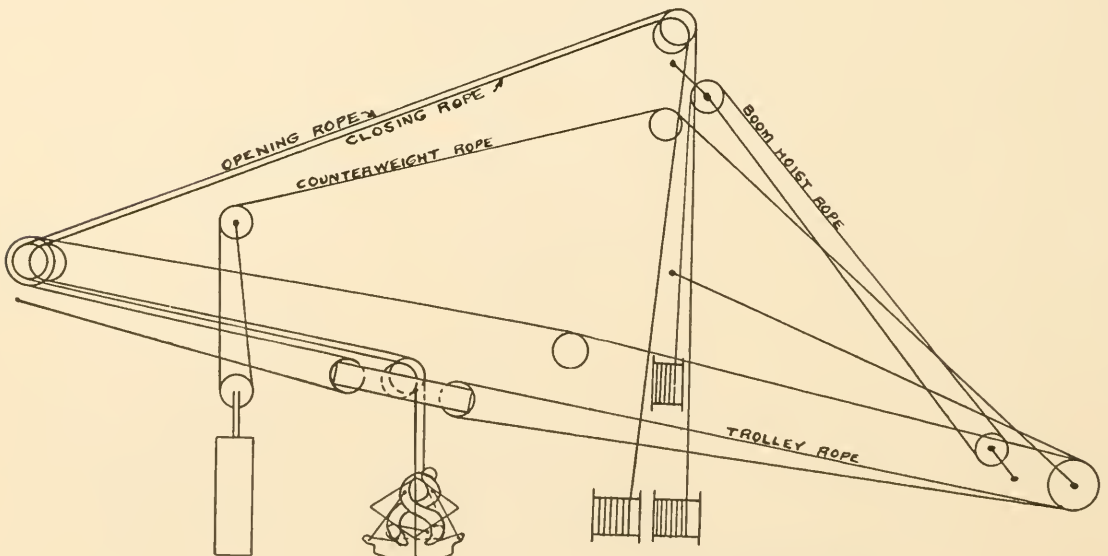
ORE UNLOADER RIG
