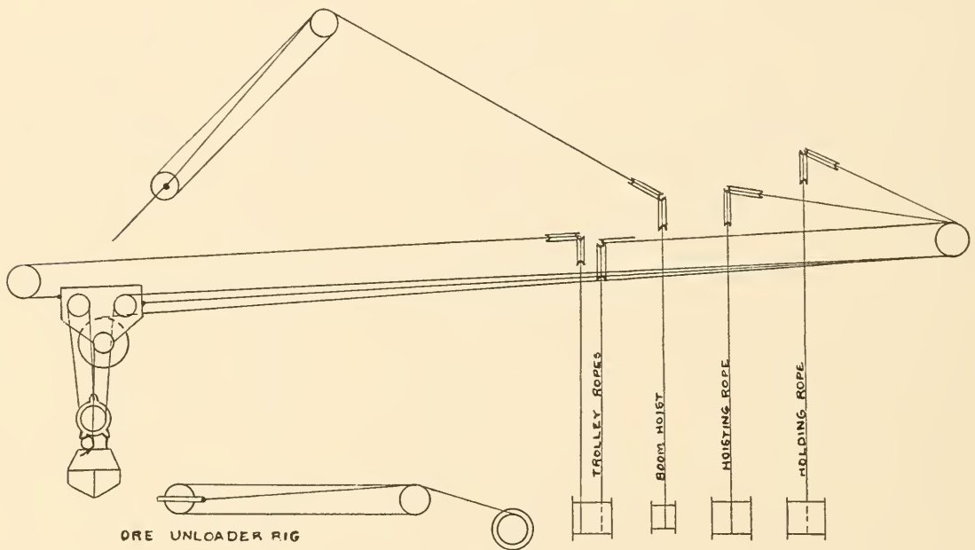
ORE UNLOADER RIG
