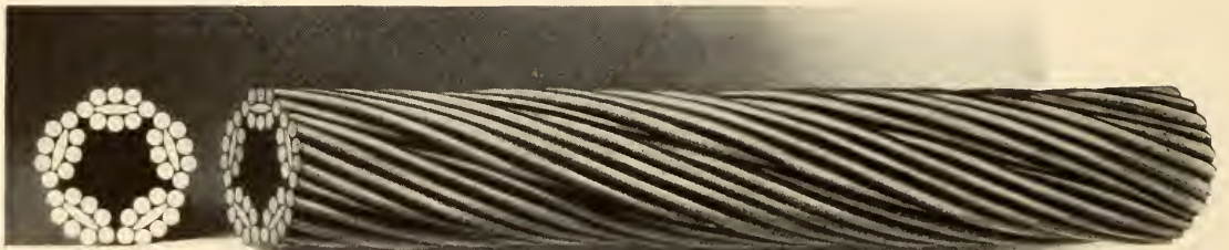
Type C—5 Strands 9 Wires—1 Hemp Core
