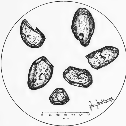
Algunos granos de monacita que integran la arena recogida en barra de Itabopoana, Río de Janeiro que le obsequiara el profesor de Mineralogía, doctor Rui Ribeiro Franco, tal como se observan a través del microscopio de polarización. Todavía hay quienes conservan su hábito prismático euhedral, que no ha podido ser borrado por la acción erosional. Dibujo del autor en preparación transitoria, n 1,552 a 15°C.
