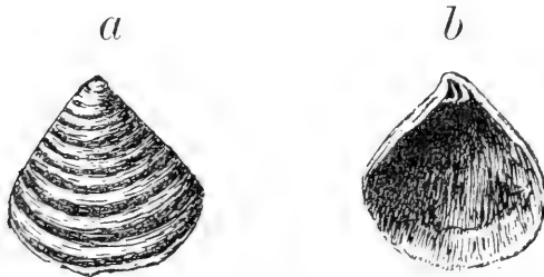
Fig. 12. Crassinella Dalli Th., valve droite, vue du côté externe (a) et interne (b): \frac{5}{1} grand. nat.
