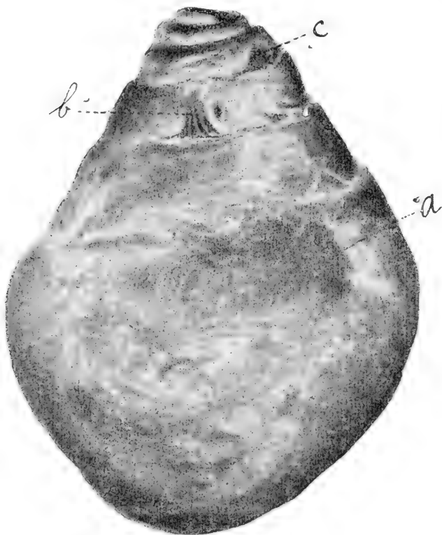
Fig. 2. — Tylostoma Rochai Th., moule interne; de grandeur naturelle.
