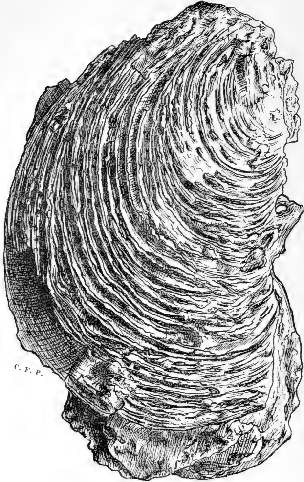
Fig. 10. — Neoinoceramus Ameghinoi Ih., vu aux \frac{3}{4} de la grandeur naturelle. Partie basale de l'étage juléen.
