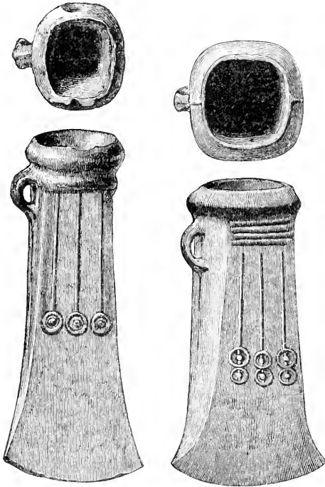
Fig. 138.—Cayton Carr. \frac{1}{2}
