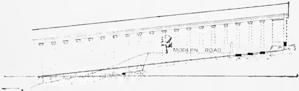
LONGITUDINAL SECTION (restored).
