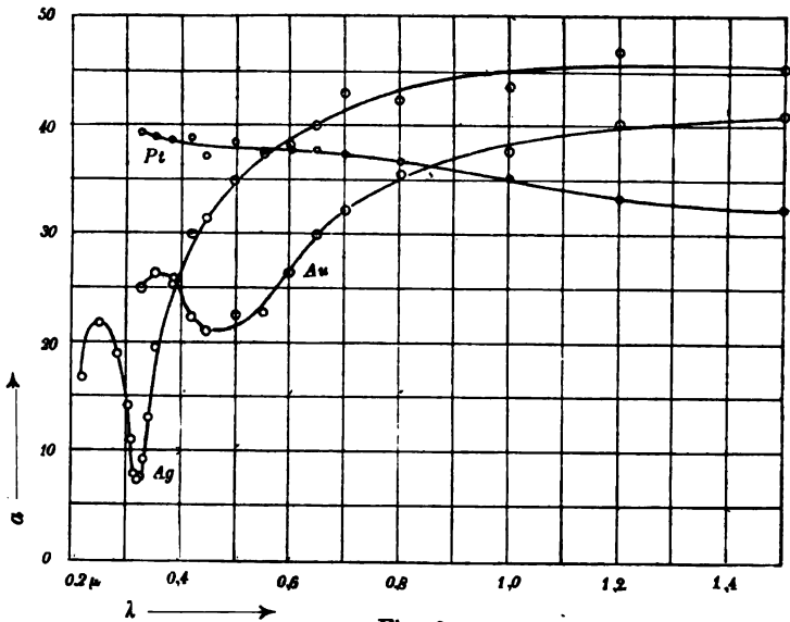
Fig. 6. Absorptionskonstante a für Ag, Au, Pt.
