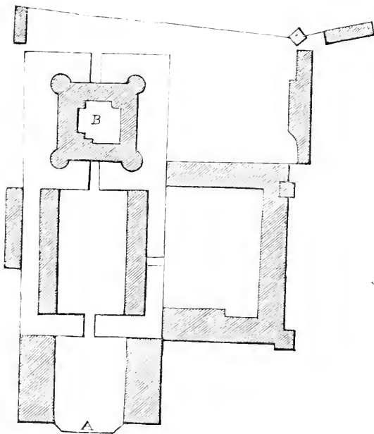
PLAN DE LA GRANDE COMMANDERIE DE VIEUX-JONGES.
