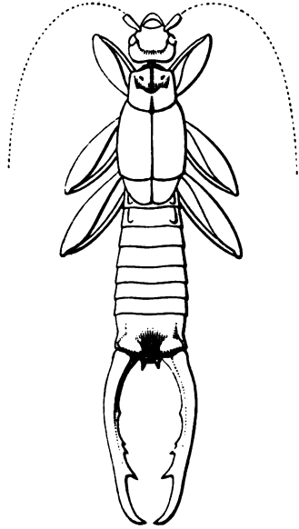
Psalidophora australica ♂.
