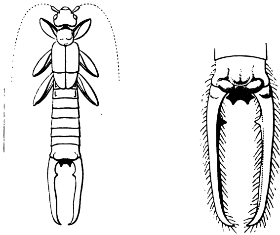
Forficula Borneensis ♂.
