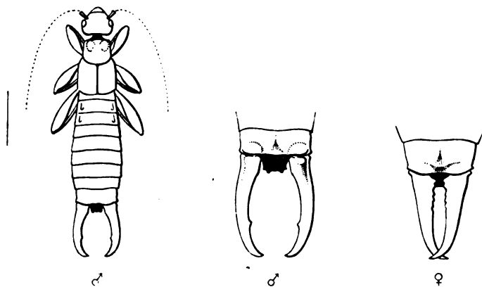
Forficula Wallacei .
