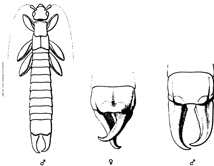
Labidura femoralis.
