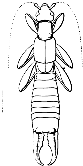
Labidurodes robustus ♂.
