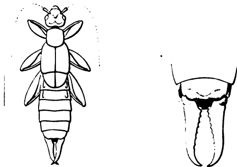
Forficula Albertisii ♀.
