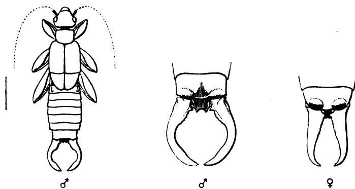
Labia Feae.
