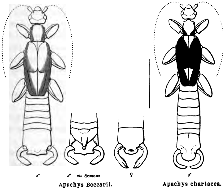
Apachys Beccarii.
