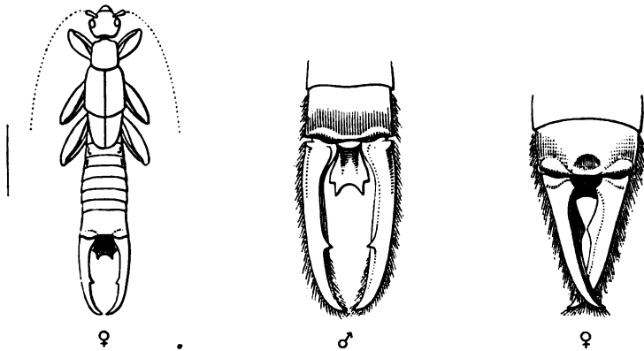
Labia pygidiata.
