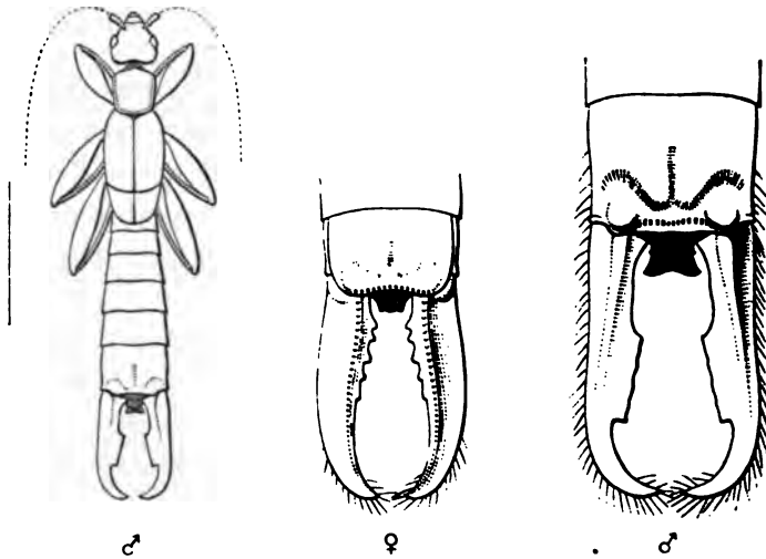
Platylabia Gestroi.
