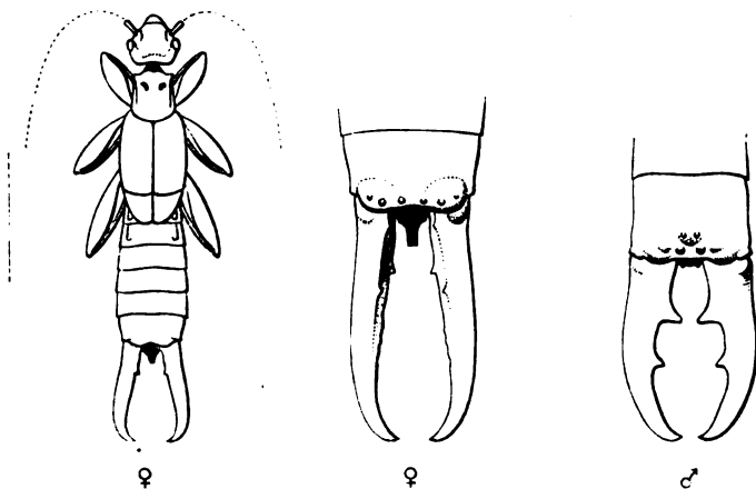
Lobophora laetior .
