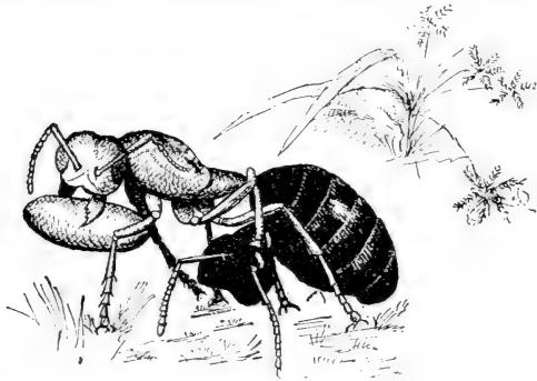
Fig. 81—SLAVE-HOLDING ANT
