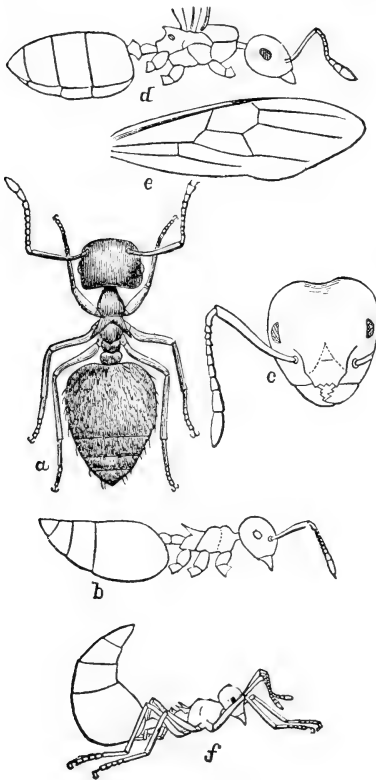
Fig. 22—CREMASTOGASTER LINEOLATA
