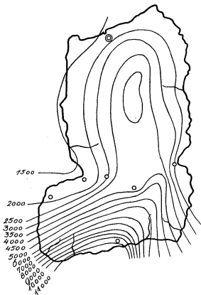
Abb. 3. Die Regenverteilung auf der Insel Fernando Poo im Jahre 1940 (nach Nosri). Die Isohyeten bezeichnen die Menge der Jahresniederschläge.
