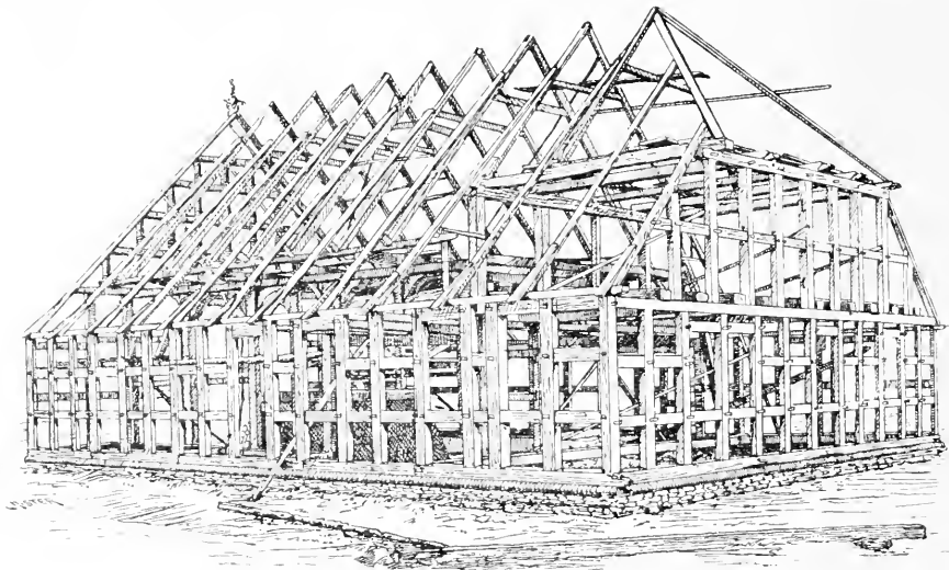
Fig. 18. Holzgerüst eines niedersächsischen Hauses.
