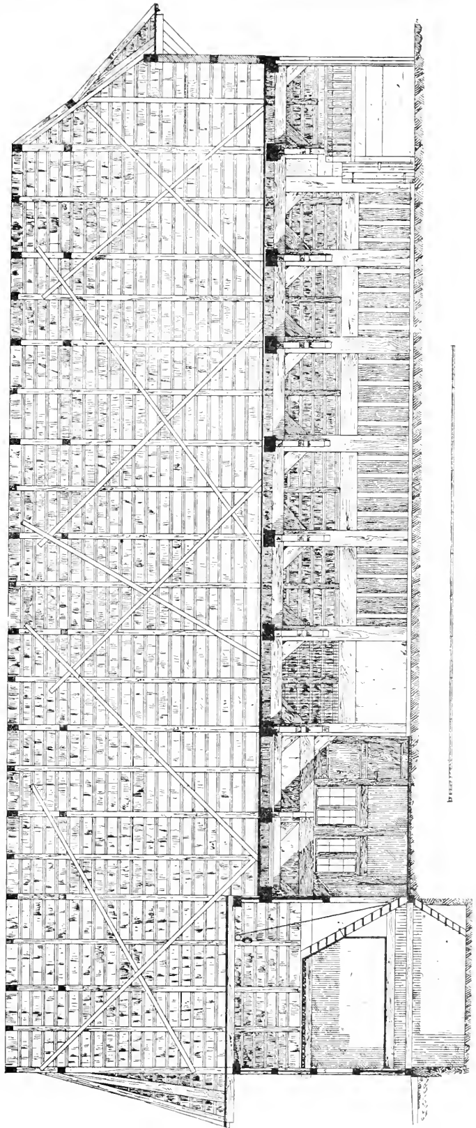
Fig. 2. Langenschnitt.
