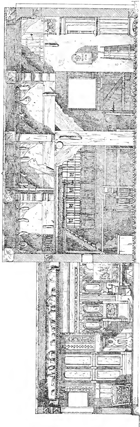
Fig. 8. Längsschnitt durch Flet und Stuben.
