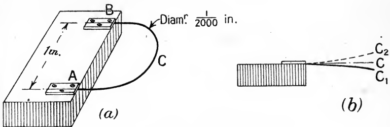
FIG. 44.—Accelerometer.
