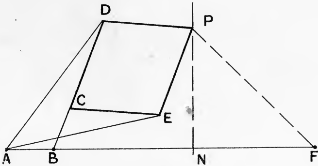
FIG. 191.—Peaucellier cell.
