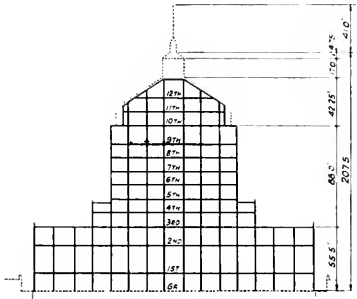
LONGITUDINAL SECTION STEEL
