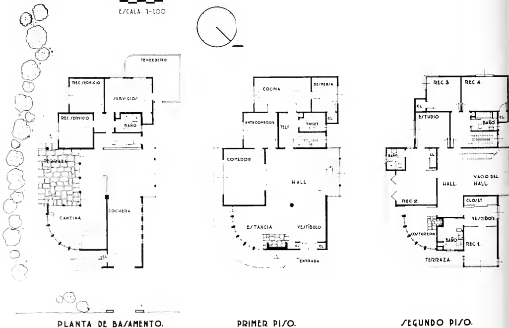
PLANTA DE BASAMENTO.
