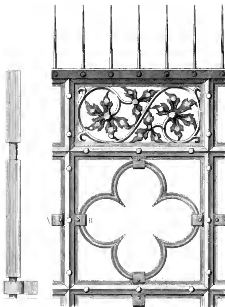
Detail à 0.10 p mètre
