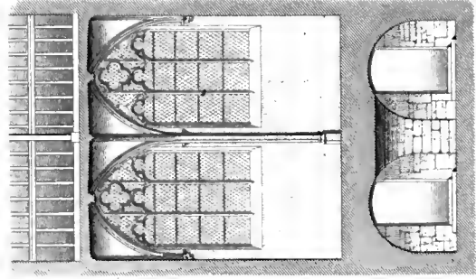
COUPE TRANSVERSALE à 0.005 P.M.
