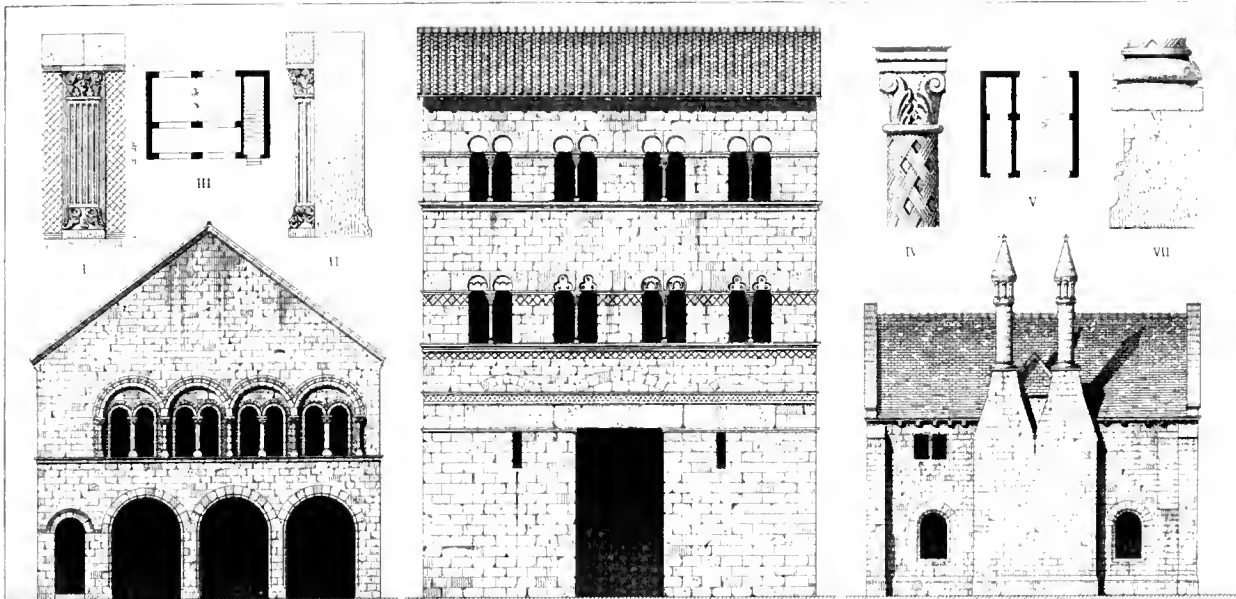
MAISON A BRANGENC
