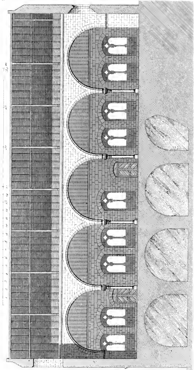
COUPRE D'ÉTAGE SUR CD
