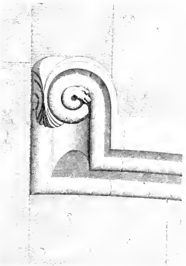
ORNICHE SUPERIEURE DE LA MAISON. A. MOULURES DE L'ARC DU BALCON MAISON. B. RETOMBES DE L'ARCHIVOÛTE PORTÉ DE LA MAISON. B. BALCON DE LA MAISON. P.
