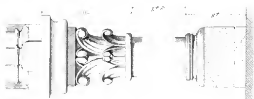
BASE ET CHÂTEAU DES COLONNES INTÉRIEURES
