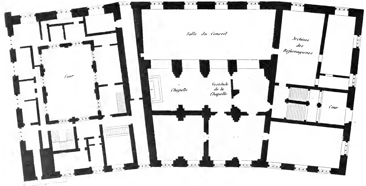
PLAN DU PREMIER ETAGE
