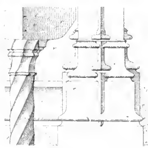
BASE DE LA PORTE E au dixieme
