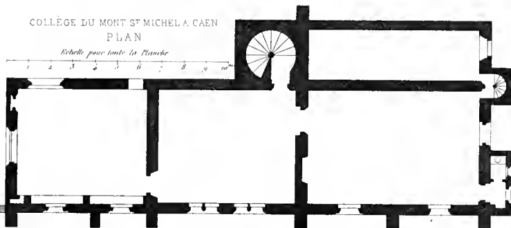
COLLEGE DU MONT ST MICHEL A CAEN
