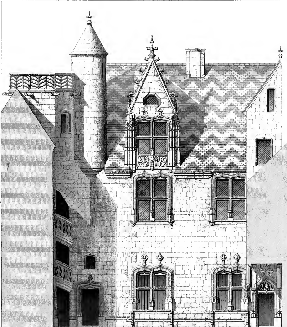
FAÇADE SUR V. X. a o o p m
