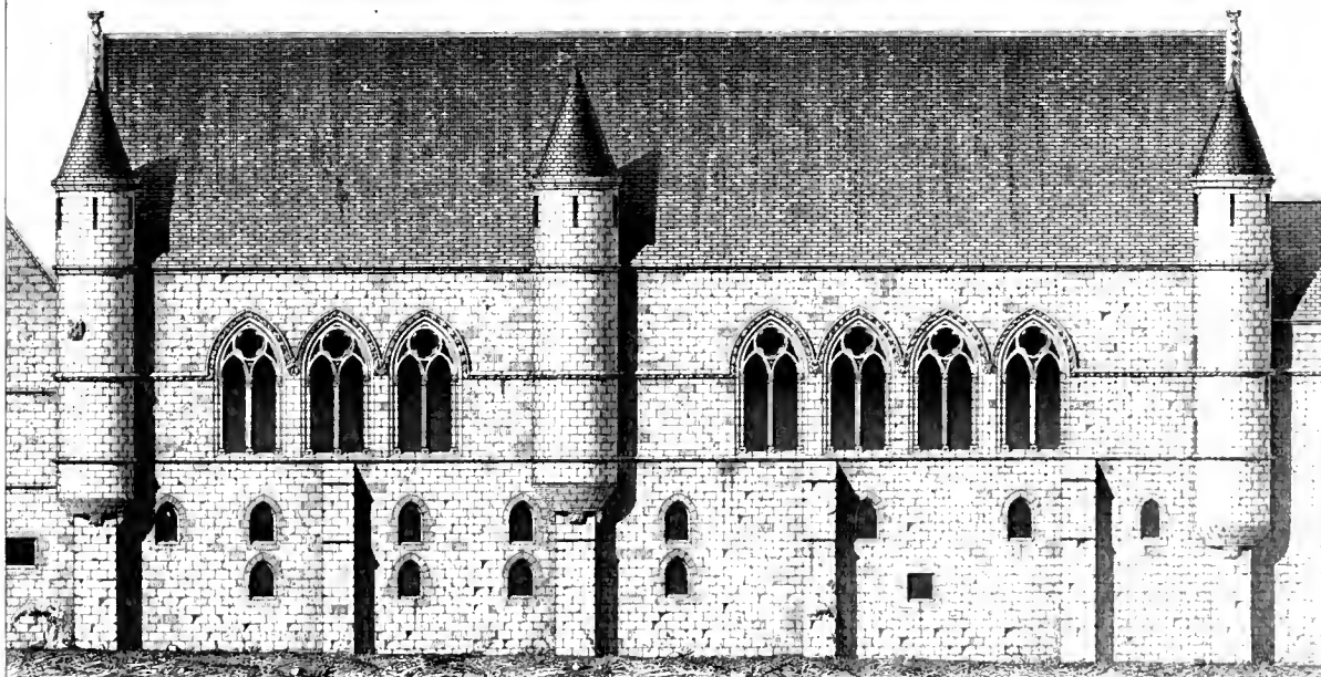
FAÇADE EXTERIEURE
