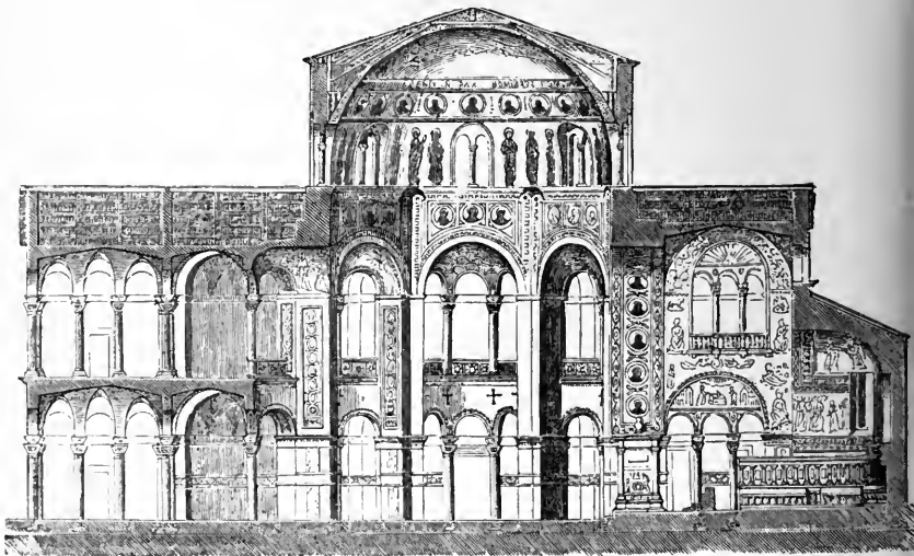
FIG. 161.—SAN VITALE AT RAVENNA. LONGITUDINAL SECTION.
