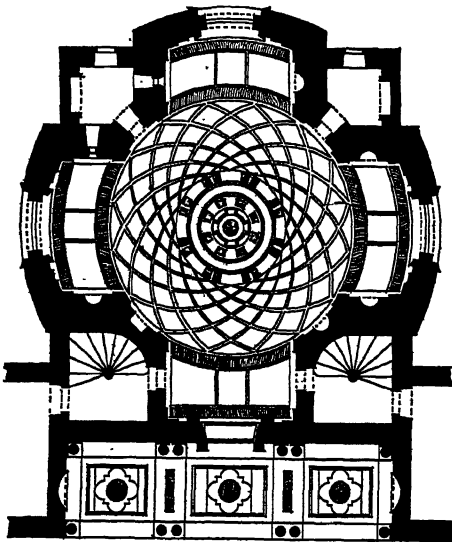
200. ANET: CHATEAU CHAPEL, BY PH. DE L'ORME. PLAN FROM DU CERCEAU. NO SCALE.
