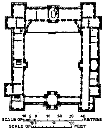
229. CHATEAU OF COULOMMIER: PLAN. FROM MAROT.
