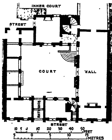
74. CAEN: HOTEL D'ÉCOVILLE: PLAN.
