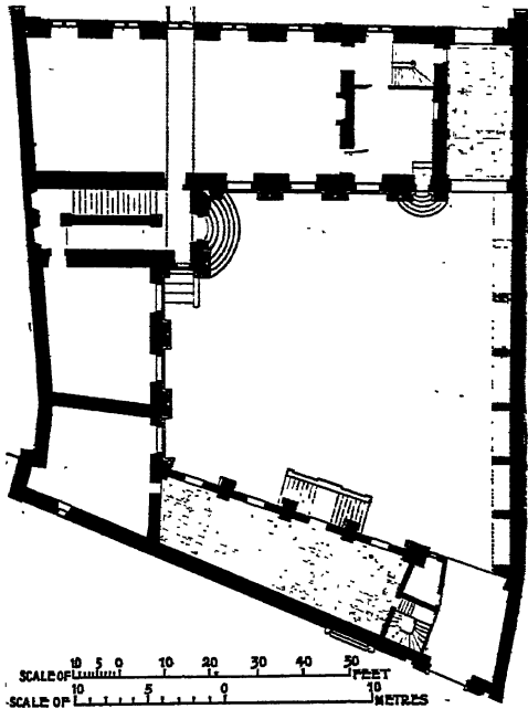
151. TOULOUSE: HOTEL D'ASSEZAT. PLAN.
